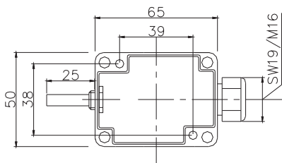
AGS 54ext Sensor AGS 54ext MODBUS
