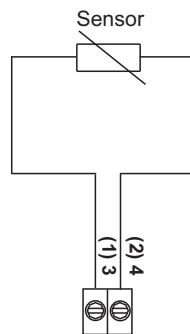
2-Leiter 2-wire
