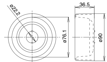
HW9Z-KG5
