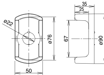
HW9Z-KG4
