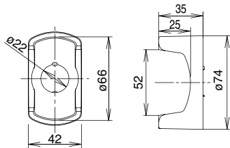
HW9Z-KG3
