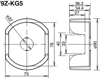
HW9Z-KG5
