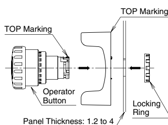
ø22 mm
