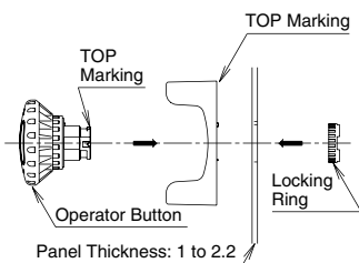
ø16 mm
