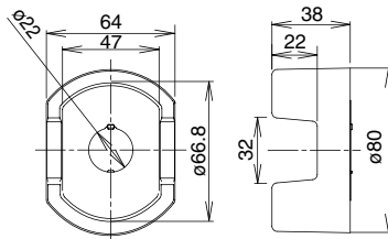
HW9Z-KG4
