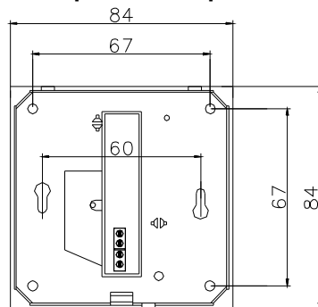
Grundplatte/Base plate
